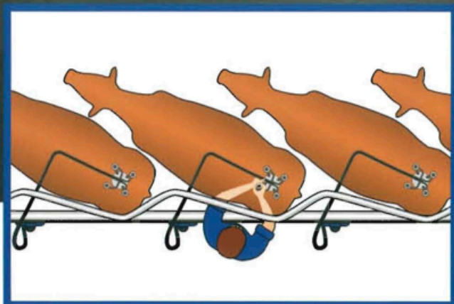
Dojnice stoja odklonené o 30° od hrany dojacej jamy. Vzdialenosť medzi kravami je 115 cm.
